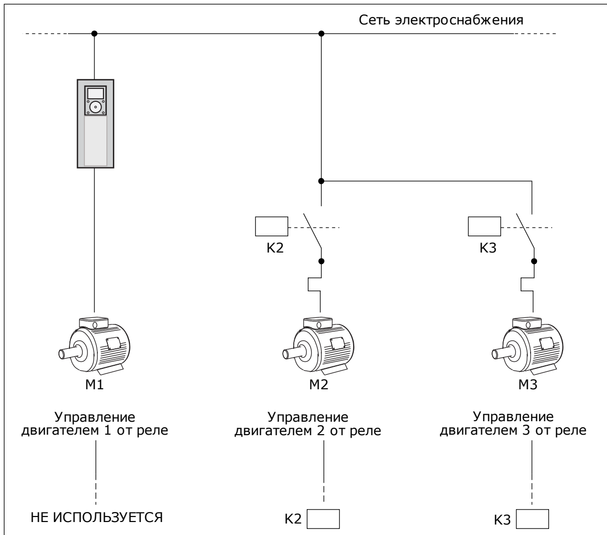
Рис. 83: Выбор 0
