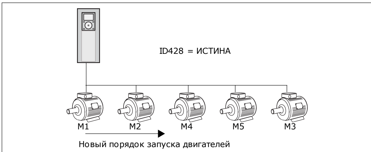
Рис. 82: Логика блокировки 3
