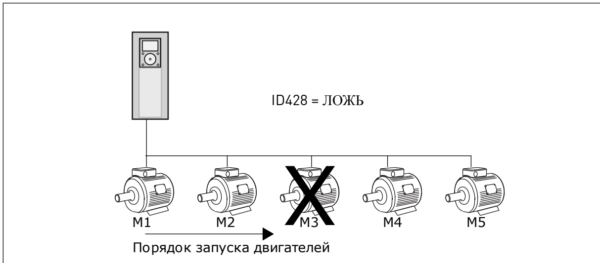
Рис. 81: Логика блокировки 2
