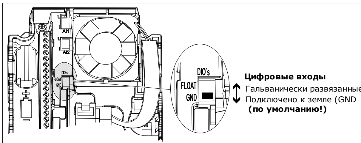
Рис. 5: DIP-переключатель
